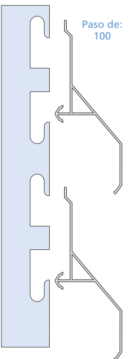
CÓD. 363024 Soporte de aluminio para fija monopared de aluminio
