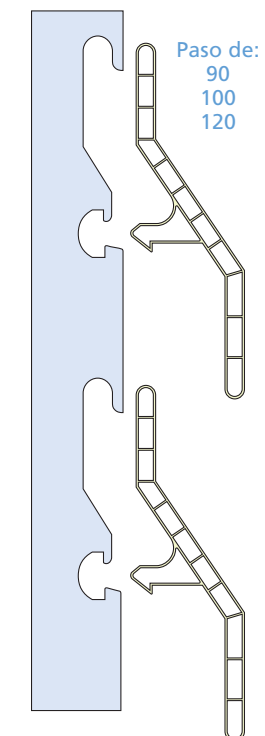
CÓD. 3630 Soporte de aluminio para doble pared de pvc
