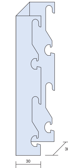
CÓD. 3630 Soporte de hierro en forma de "U" para fija monopared de pvc
