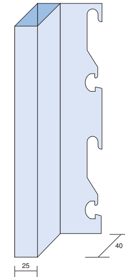
CÓD. 3630 Soporte de aluminio para doble pared de pvc
