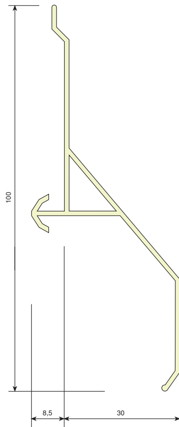
CÓD. 362510 Paño celosía Fijalux 100 monopared de pvc
