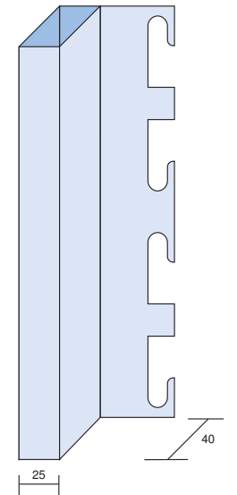
CÓD. 363024 Soporte de aluminio para fija monopared de aluminio
