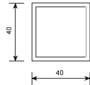
CÓD. 363056 Perfil marco de 40 x 40 mm.
