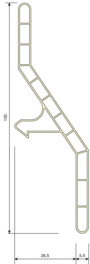
CÓD. 363012 Celosía Fijalux 100 doble pared de pvc
