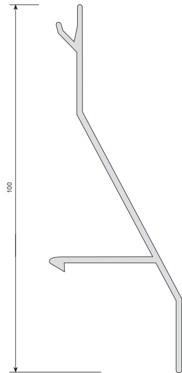
CÓD. 363011 Celosía Fijalux 100 monopared de aluminio
