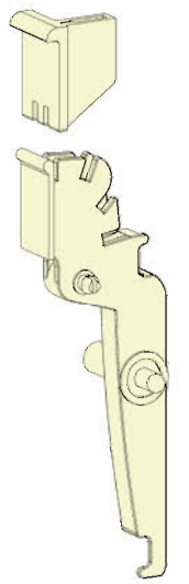
CÓD. 373703 derecha con muelle CÓD. 373705 izquierda fija Tapa mecanismo plástico
